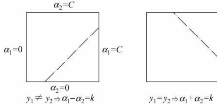
图7.8 二变量优化问题图示
