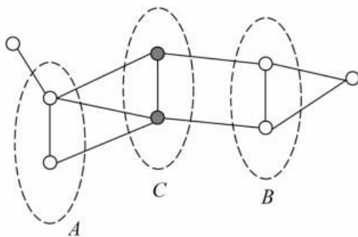
图11.2 全局马尔可夫性
