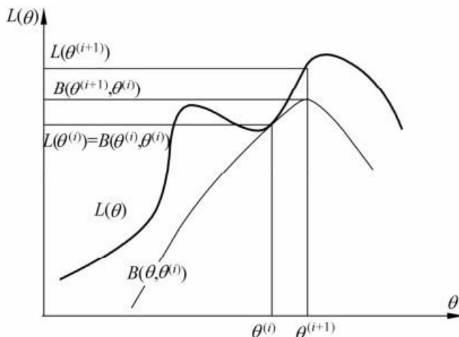
图9.1 EM算法的解释
