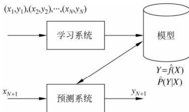
图1.1 监督学习问题
