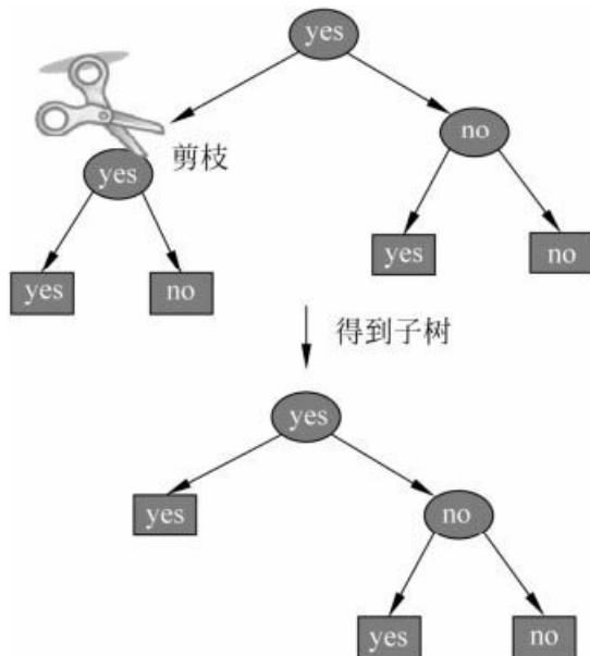
图5.6 决策树的剪枝
