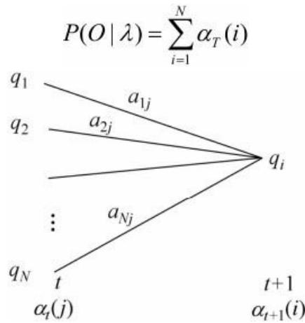
图10.1 前向概率的递推公式
