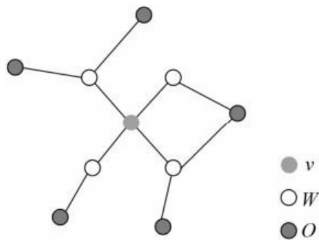
图11.1 局部马尔可夫性
