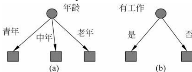
图5.3 不同特征决定的不同决策树
