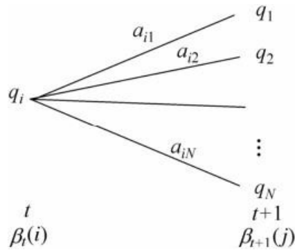
图10.3 后向概率递推公式
