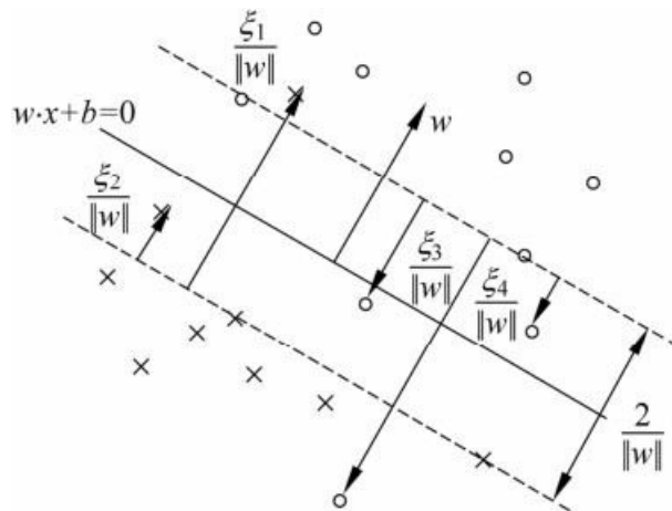
图7.5 软间隔的支持向量
