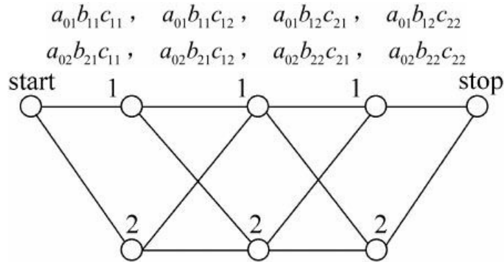
图11.6 状态路径
