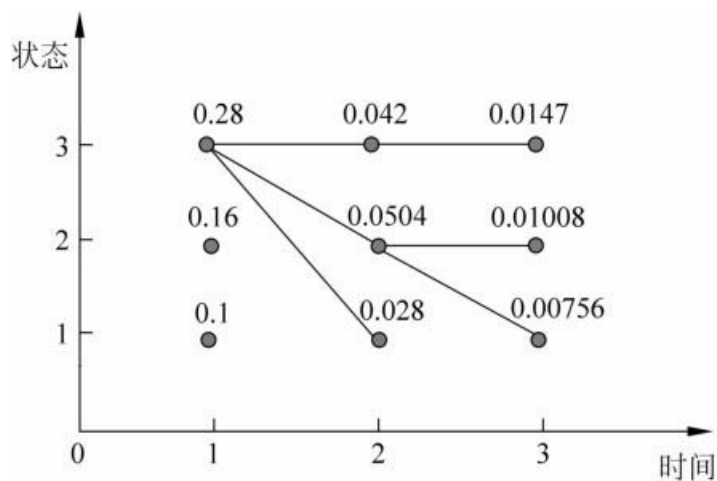
图10.4 求最优路径
