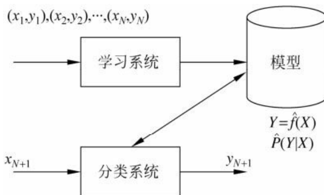
图1.4 分类问题
