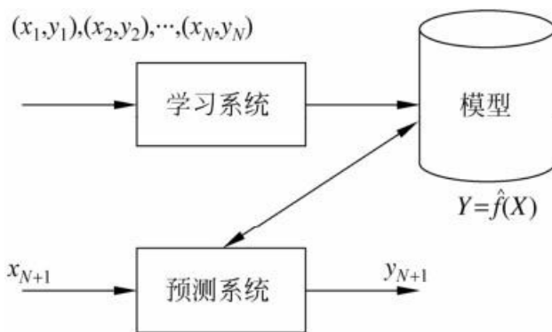
图1.6 回归问题
