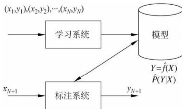
图1.5 标注问题
