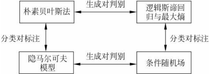
图12.1 部分模型之间的关系
