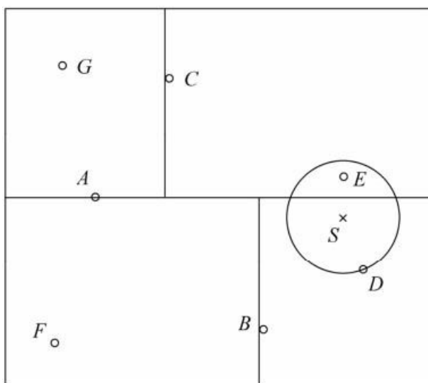
图3.5 通过kd树搜索最近邻
