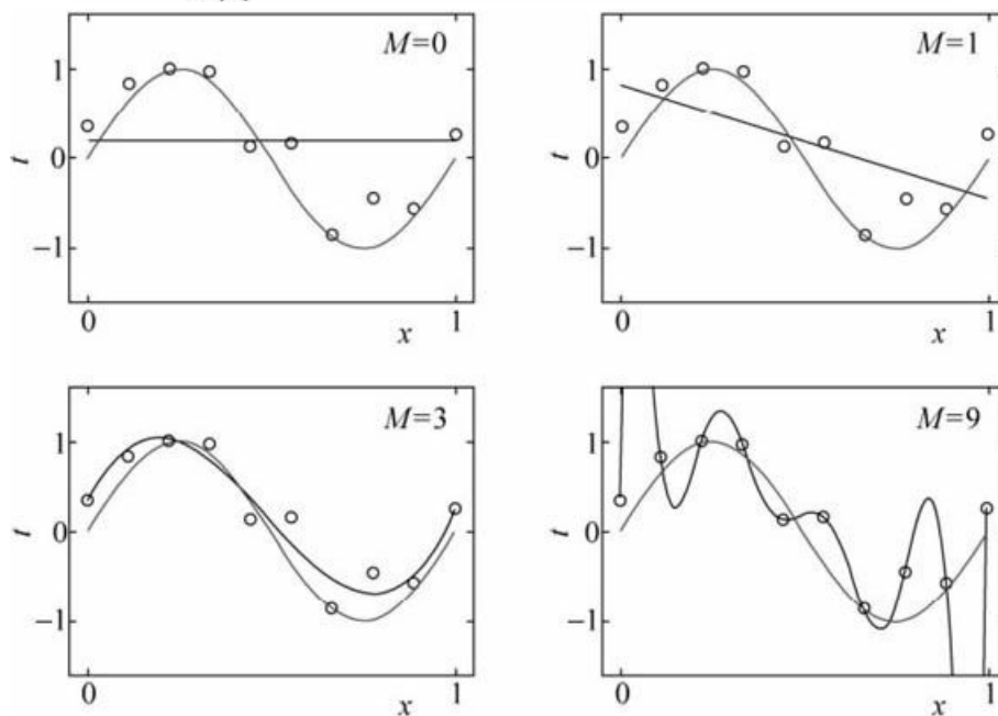
图1.2 M 次多项式函数拟合问题的例子
