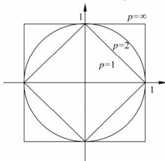
图3.2 L_p 距离间的关系
