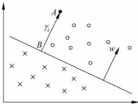
图7.2 几何间隔
