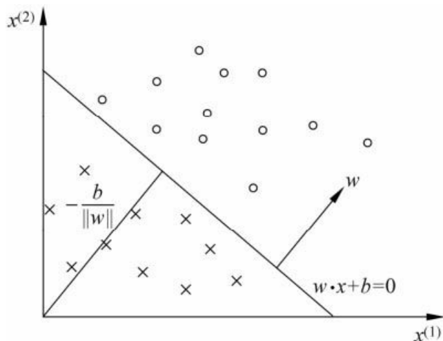
图2.1 感知机模型
