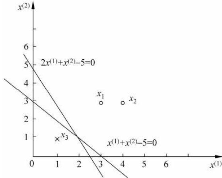
图2.2 感知机示例
