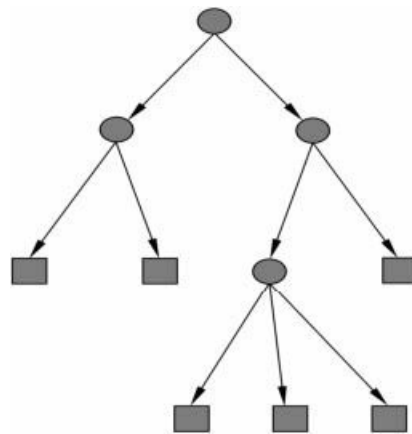
图5.1 决策树模型
