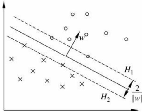
图7.3 支持向量
